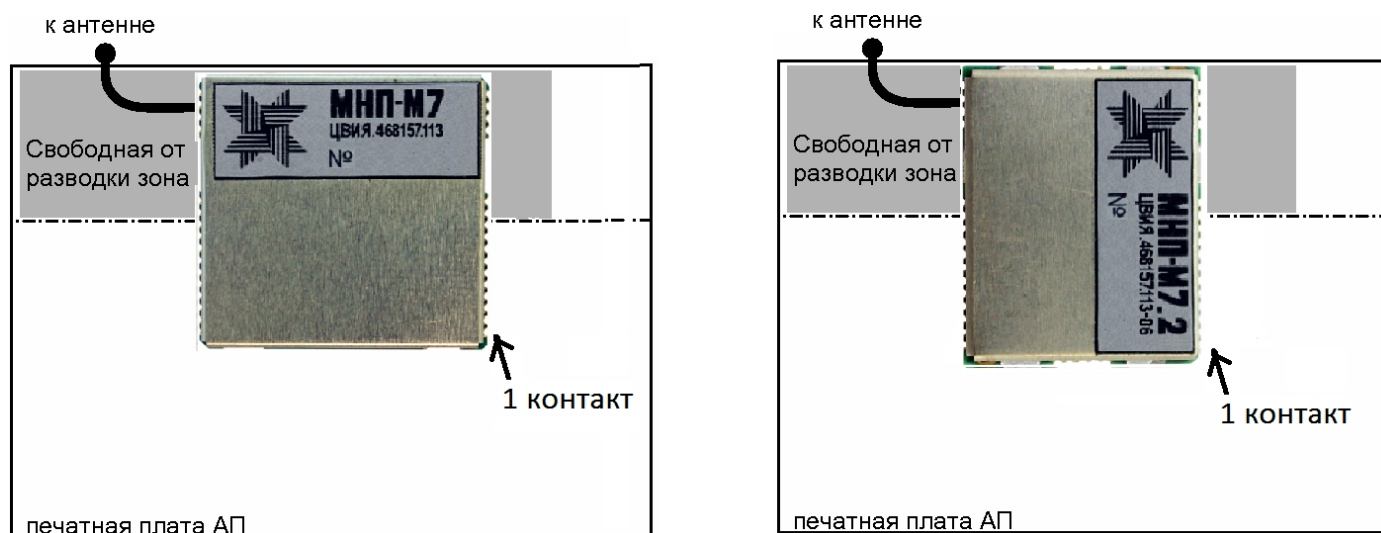
Рисунок 8 – Рекомендуемое расположение МНП-М7 (МНП-М7.2) в АП
