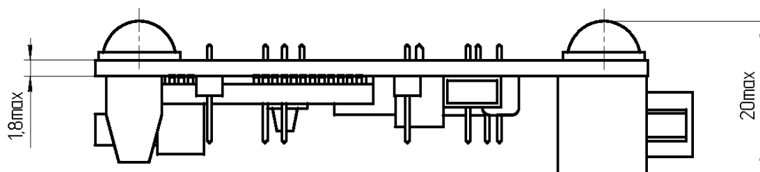
Рисунок Б.2 – Габаритный чертеж средства отладочного ЦВИЯ.468219.015-01
