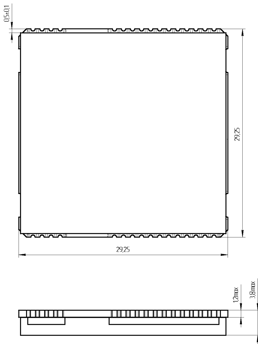
Рисунок 3 — Габаритные размеры МНП-М7 для исполнений ЦВИЯ.468157.113 и ЦВИЯ.468157.113-04
