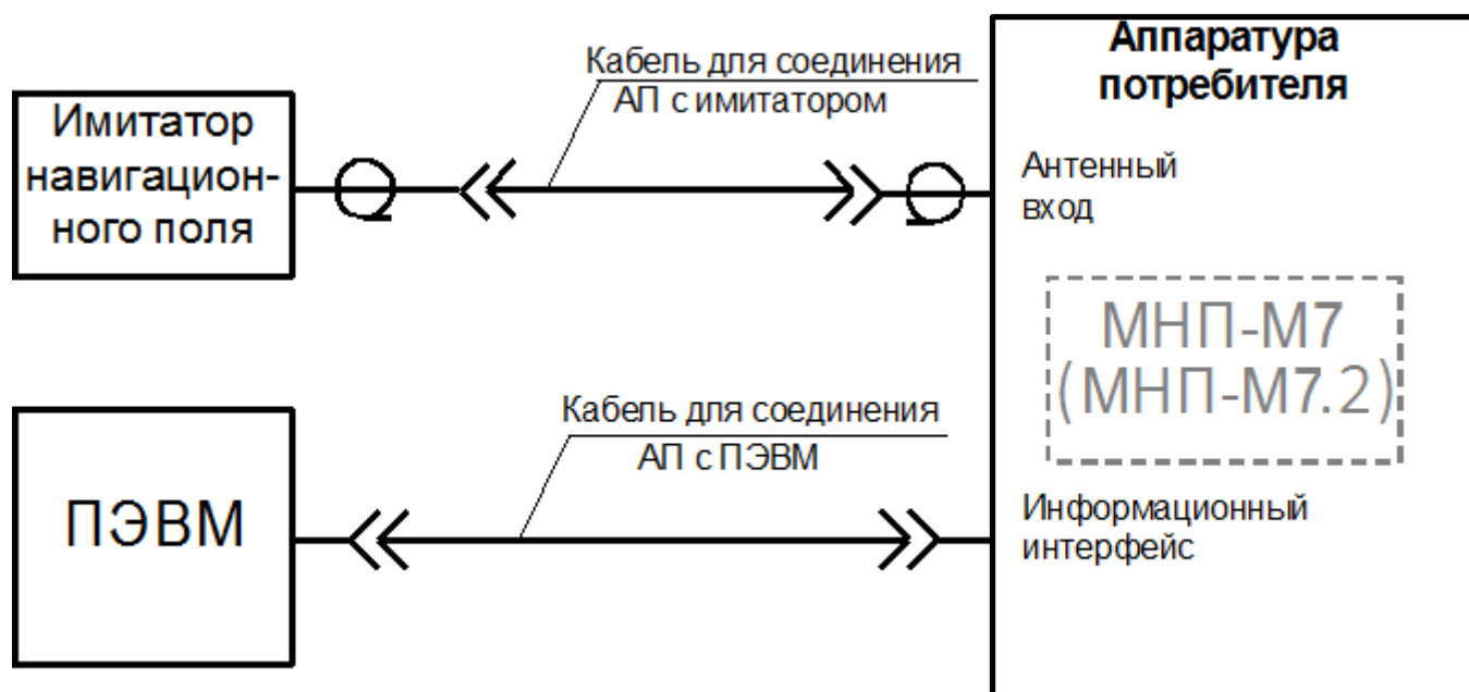
Рисунок 12 – Схема подключения МНП-М7 (МНП-М7.2) при работе с имитатором навигационного поля
