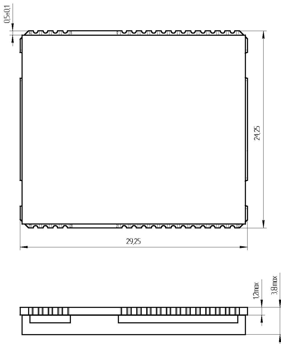
Рисунок 4 — Габаритные размеры МНП-М7.2 ЦВИЯ.468157.113-06
