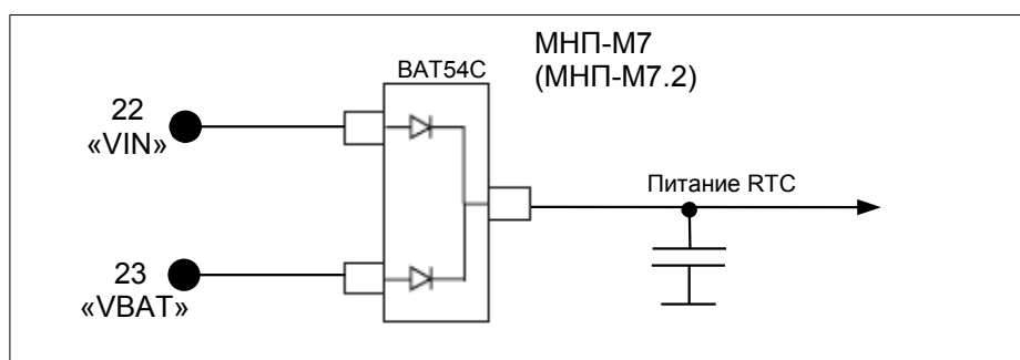
Рисунок 2 — Питание RTC в МНП-М7 (МНП-М7.2)
