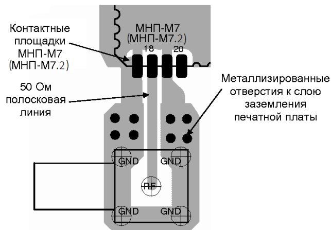
Рисунок 9 – Подключение ВЧ-соединителя к приемнику
