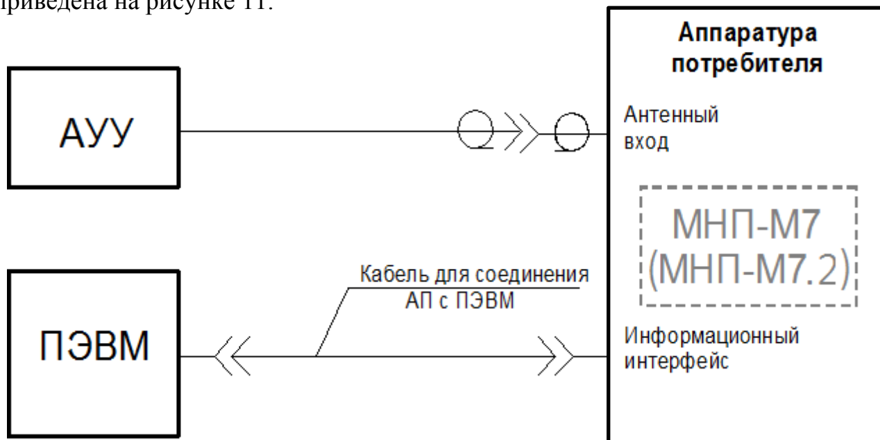
Рисунок 11 – Схема подключения МНП-М7 (МНП-М7.2) при работе по реальному сигналу
