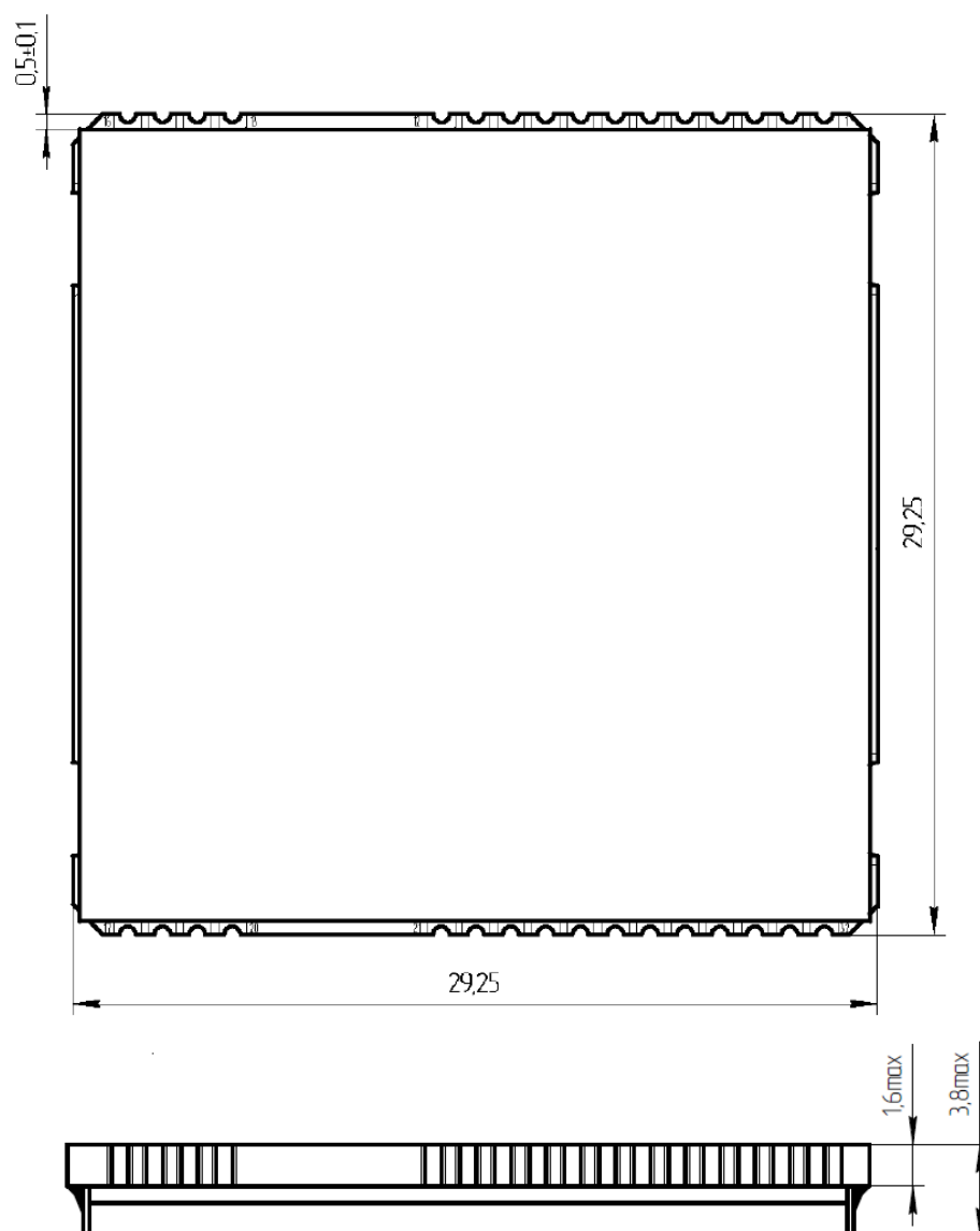
Рисунок 3 – Габаритные размеры приемника МНП-М9.1
