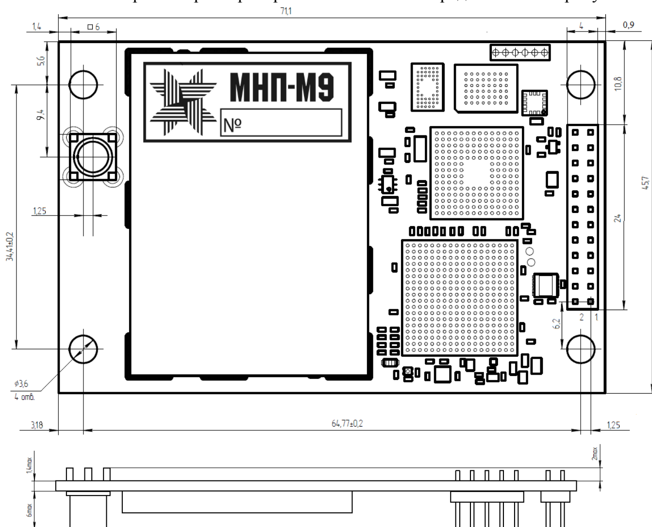
Рисунок 2 – Габаритные размеры приемника МНП-М9
