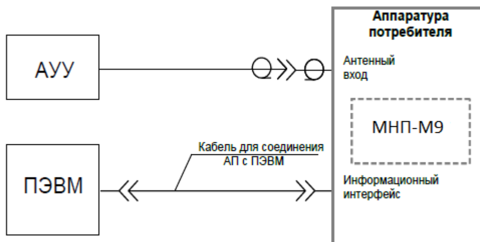
Рисунок 8 – Схема подключения приемника при работе по реальному сигналу
