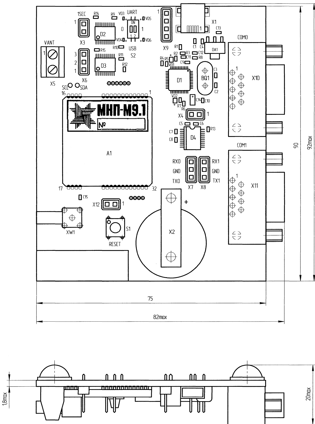
Рисунок Б.1 – Габаритный чертеж средства отладочного ЦВИЯ.468219.015-02
