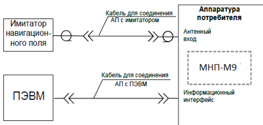
Рисунок 9 – Схема подключения приемника при работе с имитатором навигационного поля
