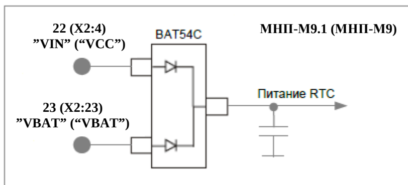
Рисунок 1 — Питание RTC в приемнике
