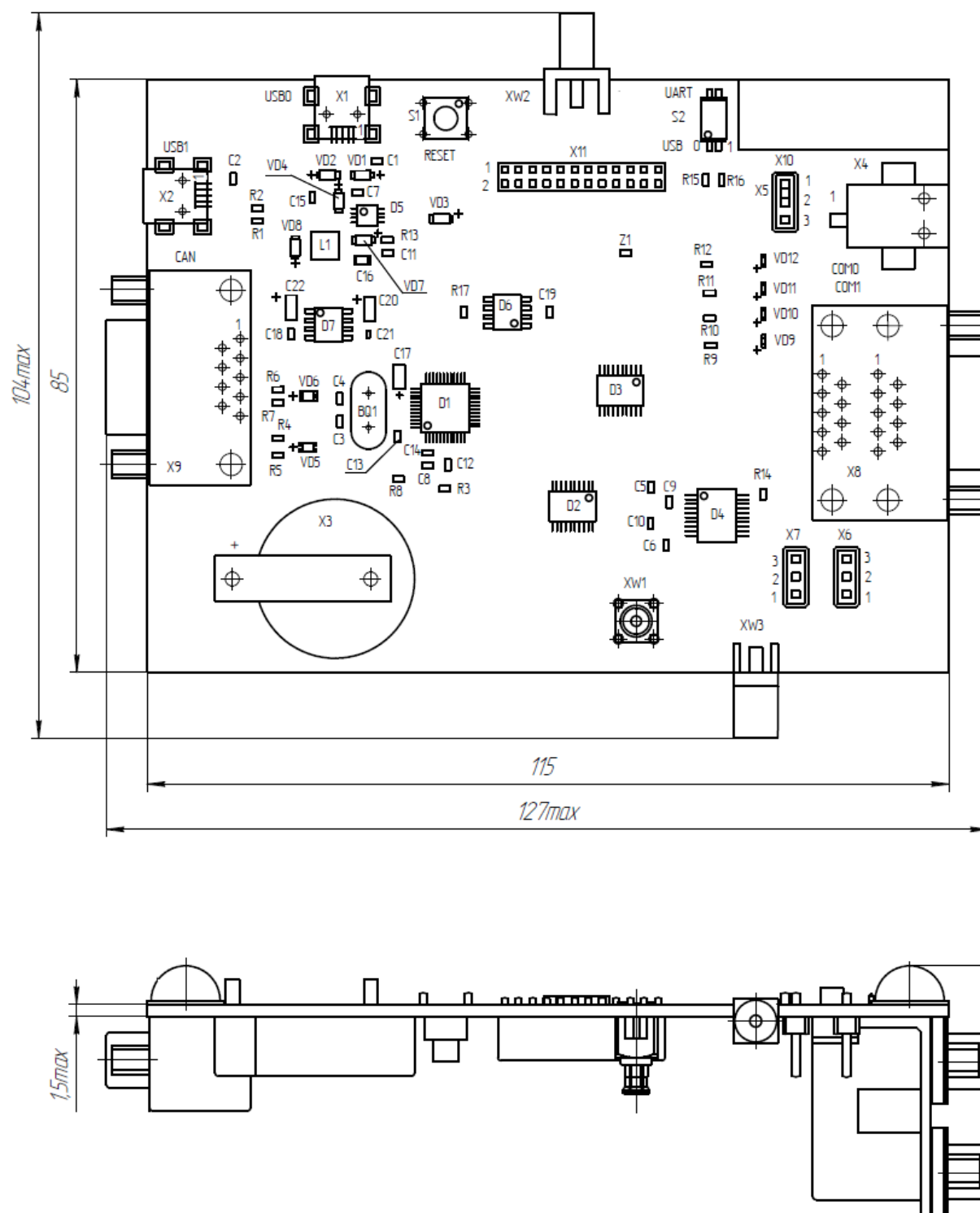
Рисунок Б.3 – Габаритный чертеж средства отладочного ЦВИЯ.468364.164
