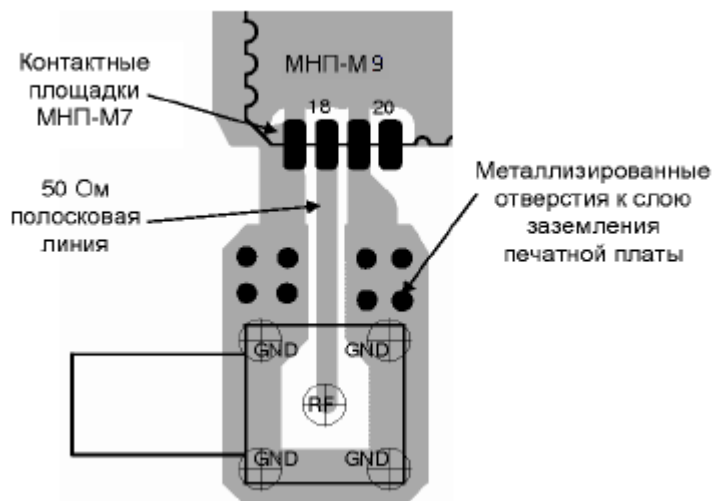
Рисунок 7 – Подключение ВЧ-соединителя к приемнику МНП-М9.1
