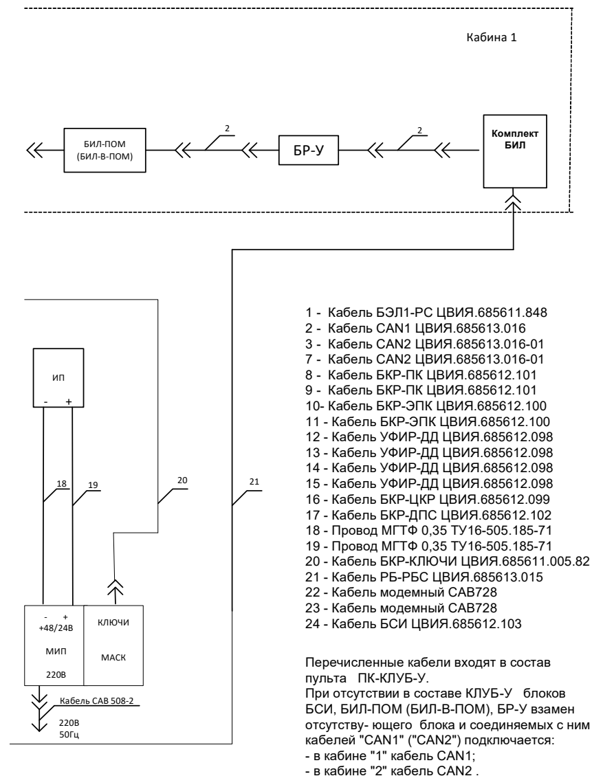
Рисунок 3 - Схема рабочего места проверки КЛУБ-У с блоком БЭЛ-УМ.
