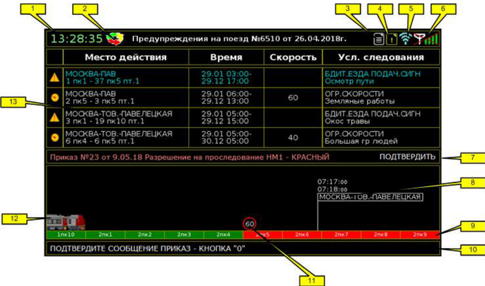
Рисунок 1.4 – Основная информация сообщений на блоке МПУЛ-И.
