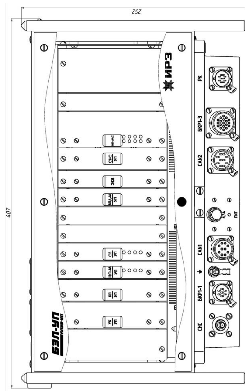
Рисунок 1 (лист 1 из 2) – Общий вид изделия
