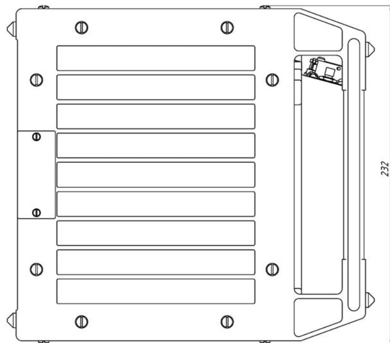
Рисунок 1 (лист 2 из 2) – Общий вид изделия
